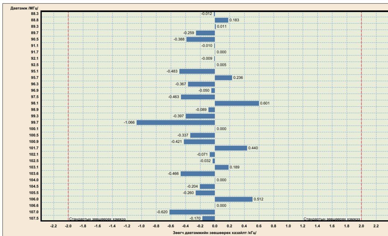
Зураг 4. Зөөгч давтамжийн зөвшөөрөх хазайлтын хэмжилтийн үр дүн
