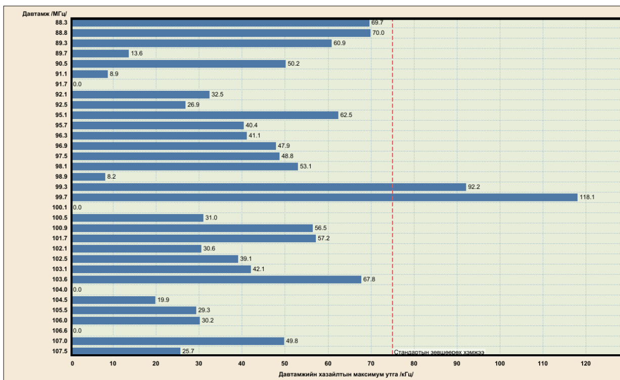
Зураг 6. Давтамжийн хазайлтын максимум утгын хэмжилтийн үр дүн
