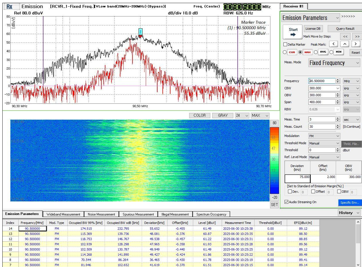
Зураг 3. Радио давтамжийн 88-108 МГц-ийн зурвасын хэмжилт
